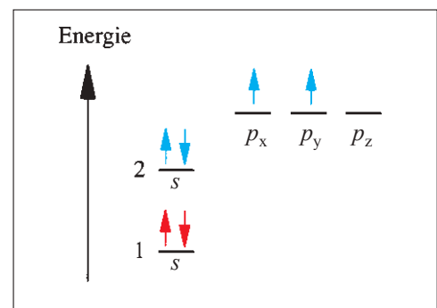
Abb. 1/2 Elektronenkonfiguration des Kohlenstoffatoms ( 1s^2 2s^2 2p^2 ).
