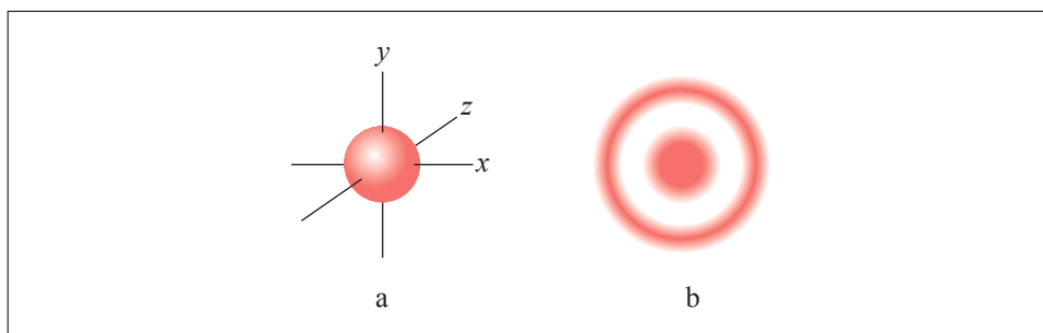
Abb. 1/3 a) Dreidimensionale Darstellung eines 1s-Orbitals. Innerhalb der Kugelgrenzen ist das 1s-Elektron mit 90%iger Wahrscheinlichkeit anzutreffen. Der Atomkern befindet sich im Zentrum. b) Querschnitt durch die Ladungswolken. Der Innenkreis stammt vom 1s-, der Außenkreis vom 2s-Orbital.
