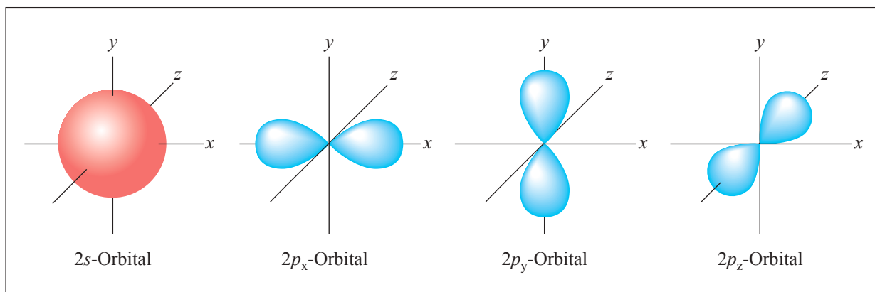
Abb. 1/4 Form und räumliche Anordnung des 2s-Orbitals und der 2p-Orbitale.
