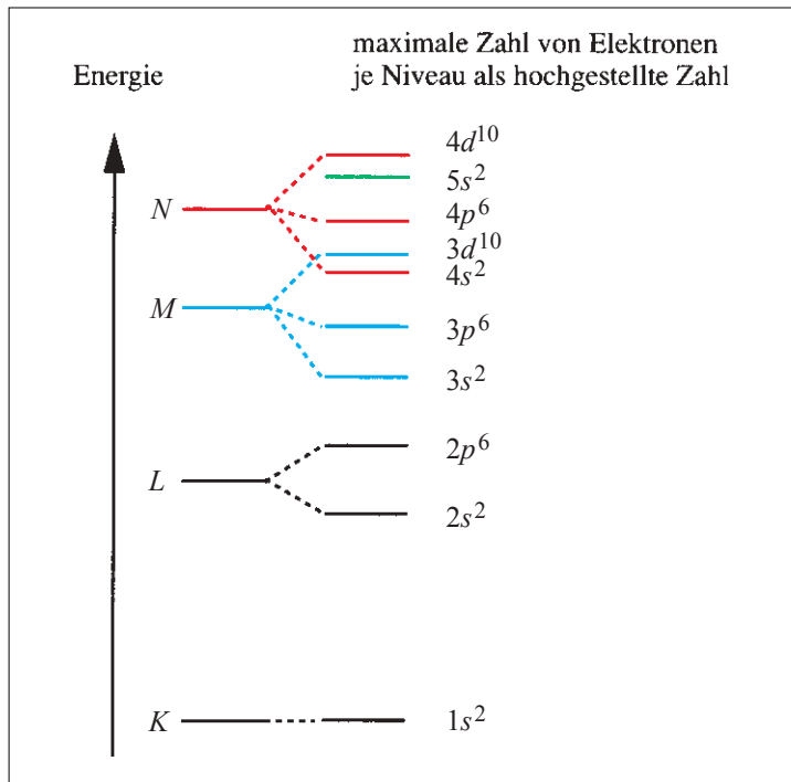
Abb. 1/1 Energieniveauschema der Elektronenhülle mit Kennzeichnung der Schalen und der Unterniveaus.
